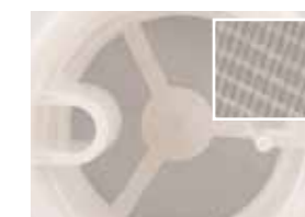
水箱过滤器端口直径：0.5mm
